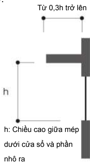
Hình A.1 - Phần che chắn nhô ra
